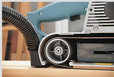
Anschluß für die Staubabsaugung (LB31E).
